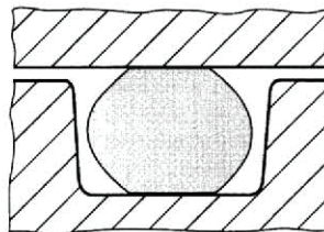
verpresster O-Ring in ohne Systemdruck
