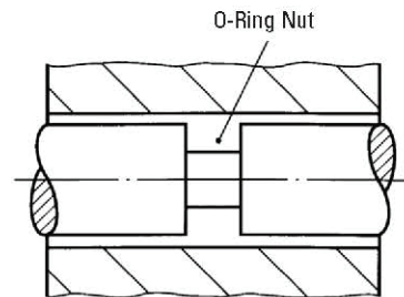
verpresster O-Ring in ohne Systemdruck
