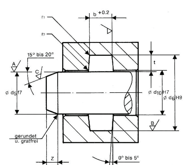
Einbaum Stangendichtung (Hydraulik + Pneumatik)
