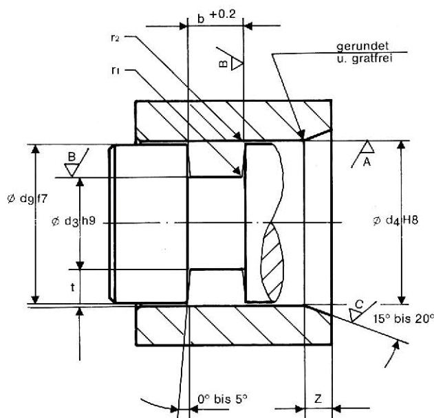
Einbaum Kolbendichtung (Hydraulik + Pneumatik)
